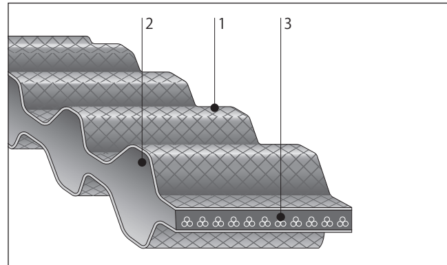
1. 歯布 2. 歯ゴム 3. 心線
