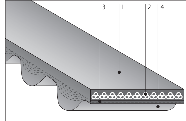
1. 背ゴム 2. 心線 3. 特殊繊維 4. 歯ゴム
