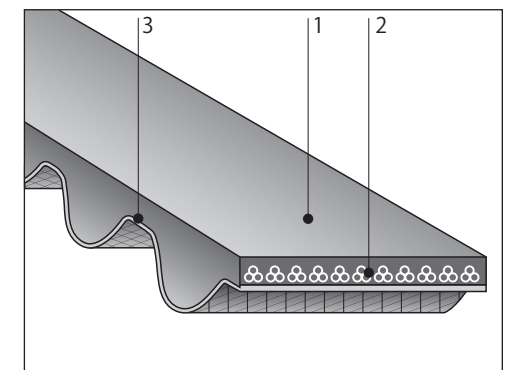
1. 背ゴム 2. 心線 3. 歯布
